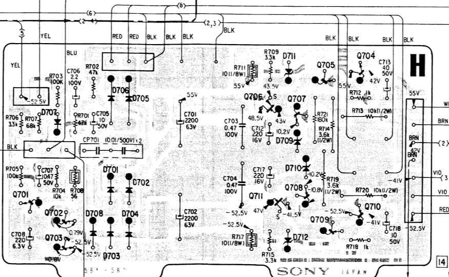
【POWER SUPPLY (A) BOARD】
