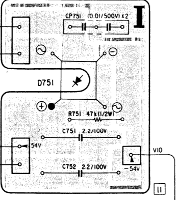
【POWER SUPPLY (B) BOARD】
