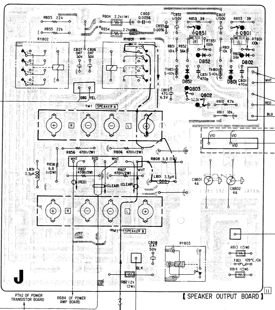
【SPEAKER OUTPUT BOARD】
